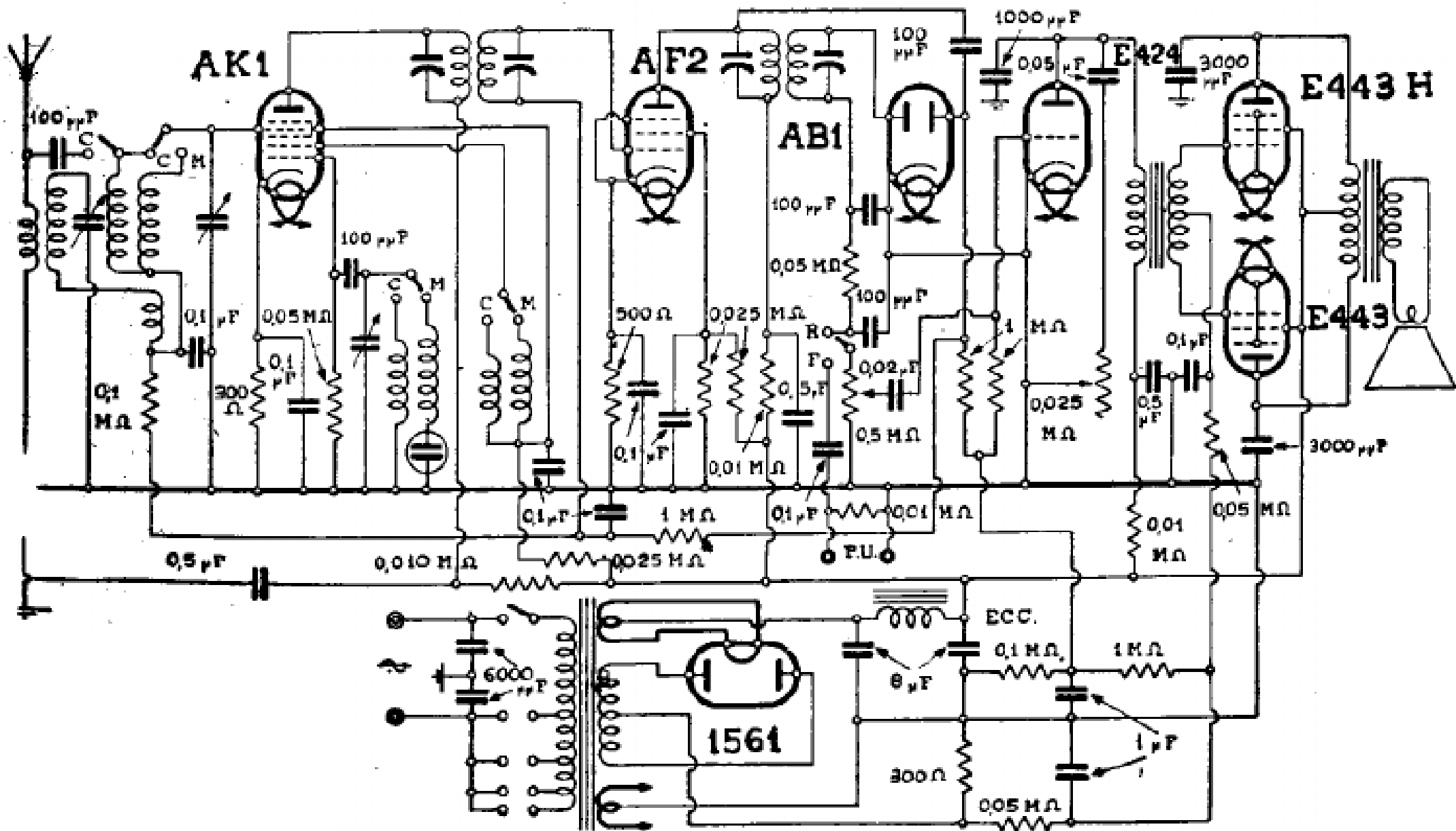
RADIO LAMBDA - MOD. « E 427-C.M. »
